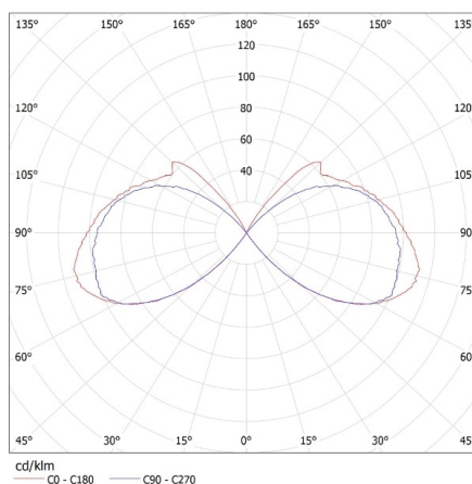
KANLUX S.A. (kat 14936) TANO G4 SMD-WW / LDC (Polar)
