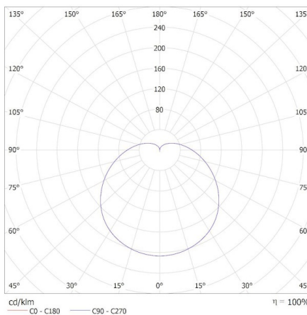
KANLUX S.A. (kat 36679) IQ-LED A60 11W-WW / Krzywa rozsyłu światła (biegunowo)
